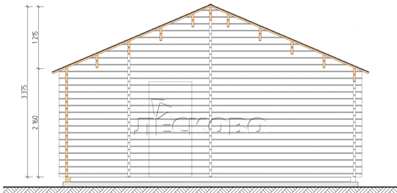
Разрез
